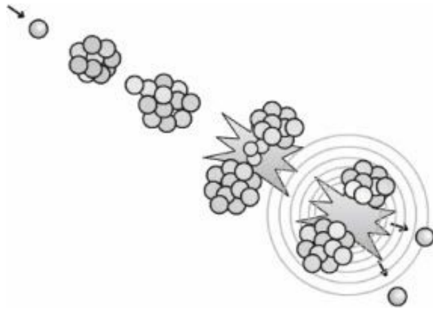
核裂变
