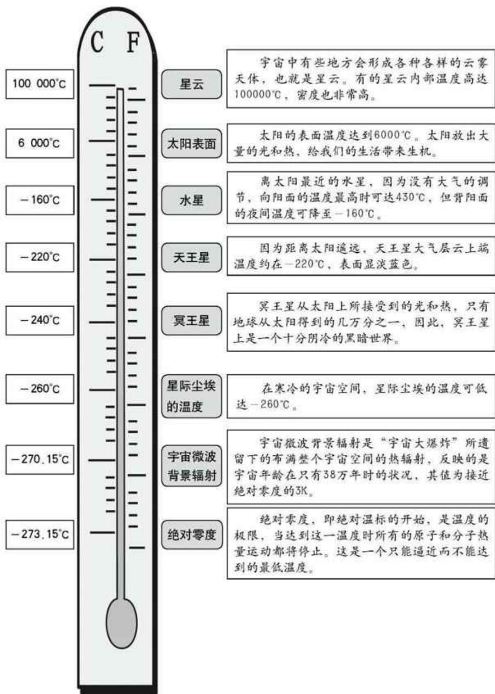
宇宙温度计
